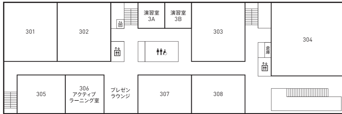
3F 大講義室304 Large Lecture Room 中講義室301・303・305・307・308 Medium Lecture Room 演習室3A・3B Seminar Room アクティブラーニング室306 Active Learning Room プレゼンラウンジ Presentation Lounge
